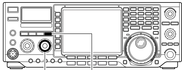
[NR](control) [NR](switch)
